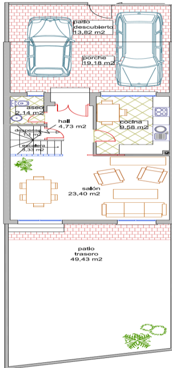
P. BAJA PARCELA 28
